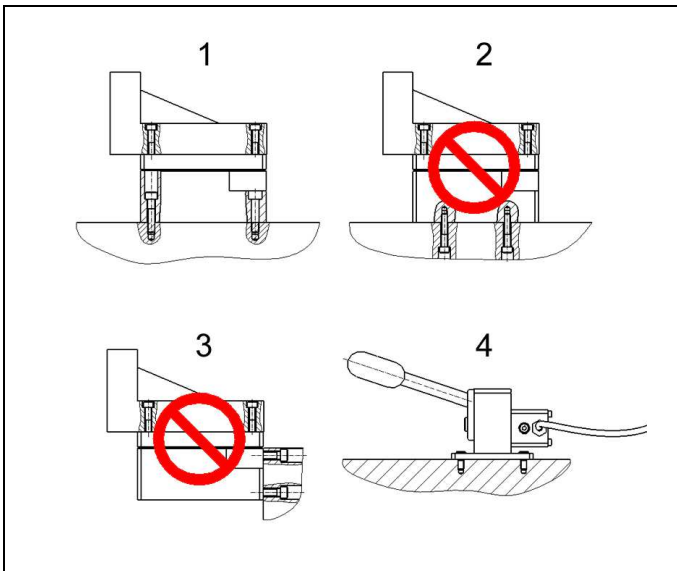
Abb. 3: Mögliche Prinzipien der Befestigung
