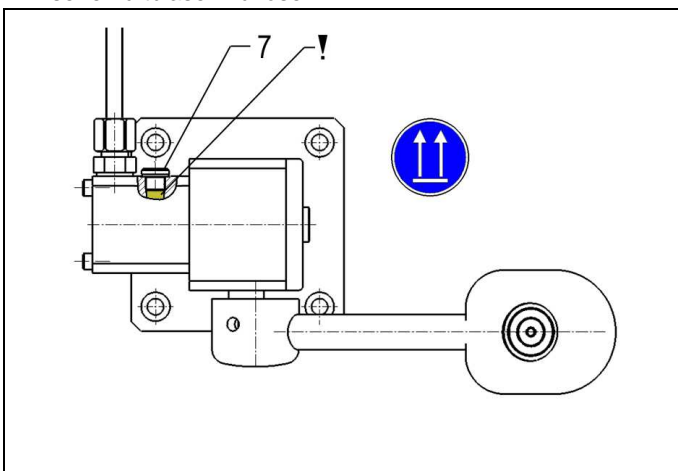
Abb. 6: Ausrichtung zur blasenfreien Montage der Verschraubung
