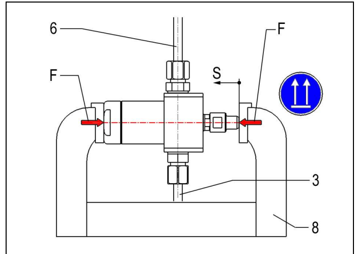
Abb. 7: Ausrichtung zur blasenfreien Montage der Verschraubung
