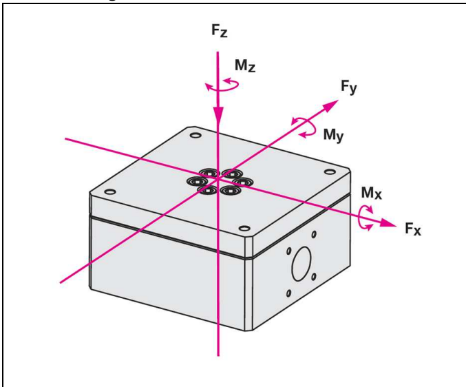
Abb. 8: Achsen der eingeleiteten Kräfte und Drehmomente
