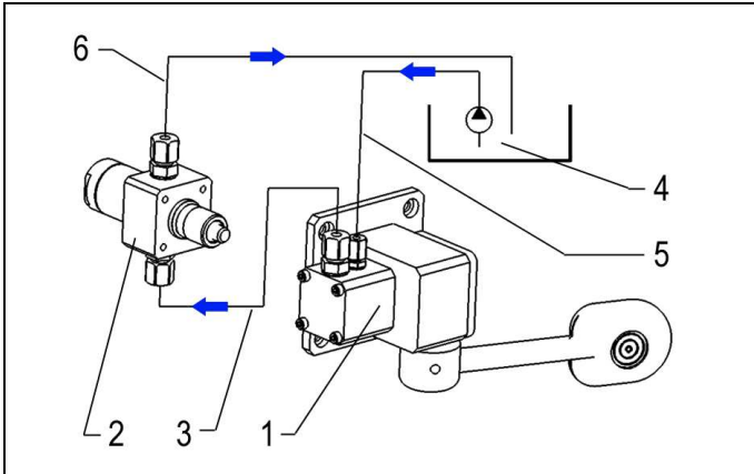
Abb. 5: Prinzipskizze zur Entlüftung der Indexierung
