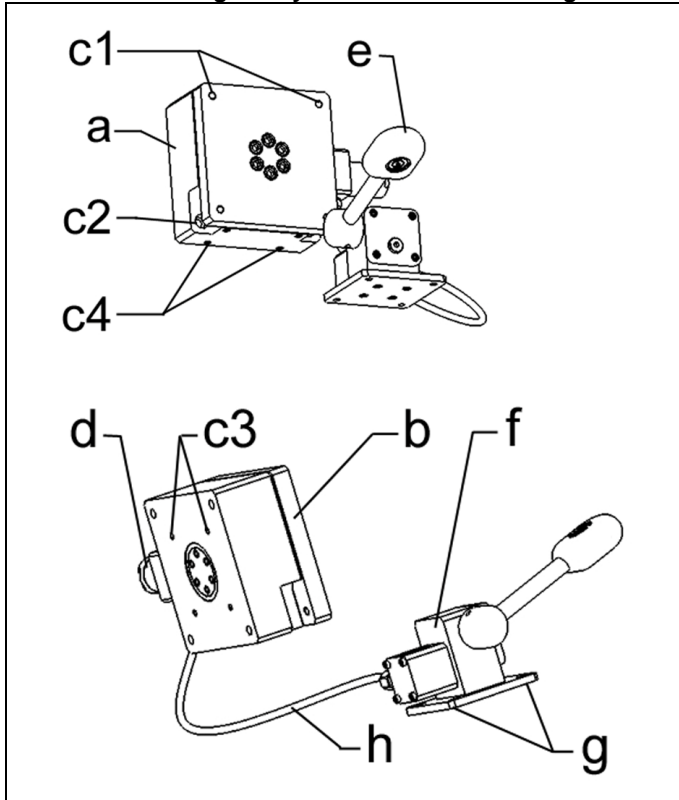
Abb. 1: Komponenten
