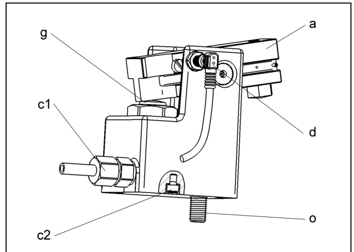
Abb. 1: Komponenten
