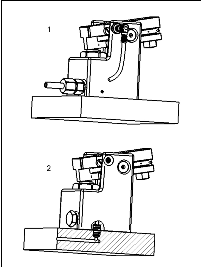
Abb. 2: Befestigungsmöglichkeiten
