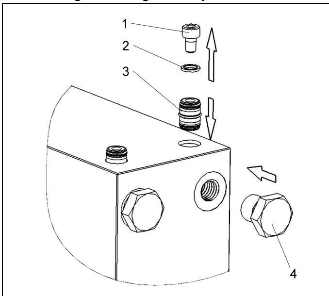
Abb. 4: Beispiel der Vorbereitung für leitungslose Hydraulikanschlüsse mittels Steckverbindung
