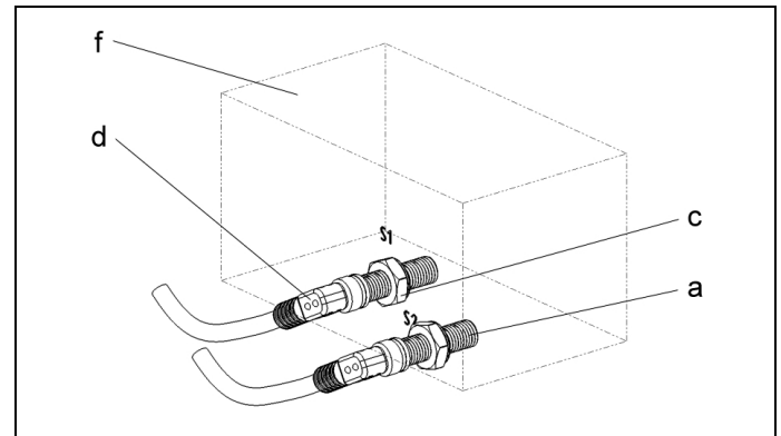
Abb. 6: Komponenten (Prinzip Einbau in einer Spannpratze)
